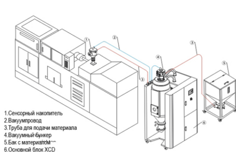
Для обслуживания одной машины: двухступенчатая конвейерная система (стандарт)
