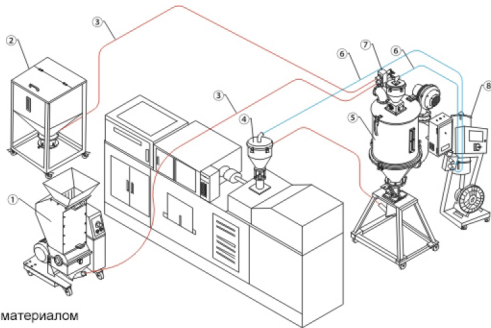
Модель 900G2 (двухступенчатый конвейер)
